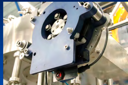
La vitesse de pose des bouchons est synchronisée avec la cadence de la machine
